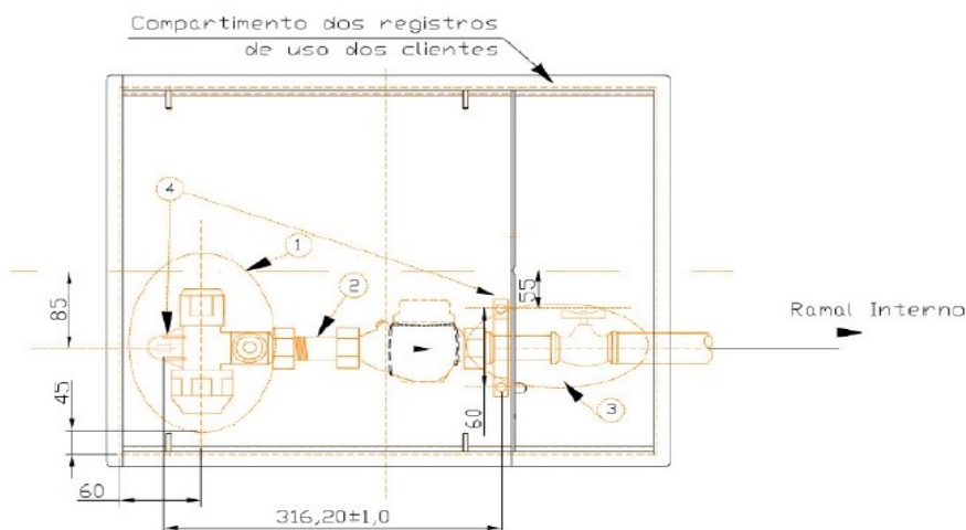
Figura 1 – Desenho esquemático de um dispositivo de medição
