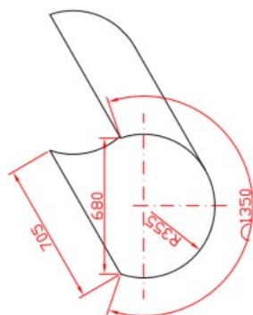
CHAPA PERFURADA SUPERIOR
