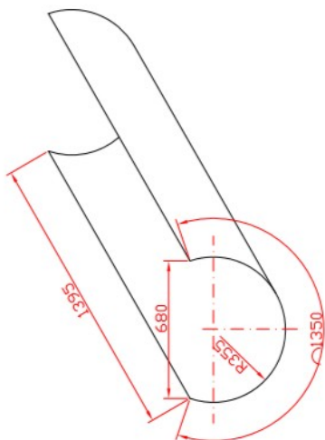
CHAPA PERFURADA INFERIOR
