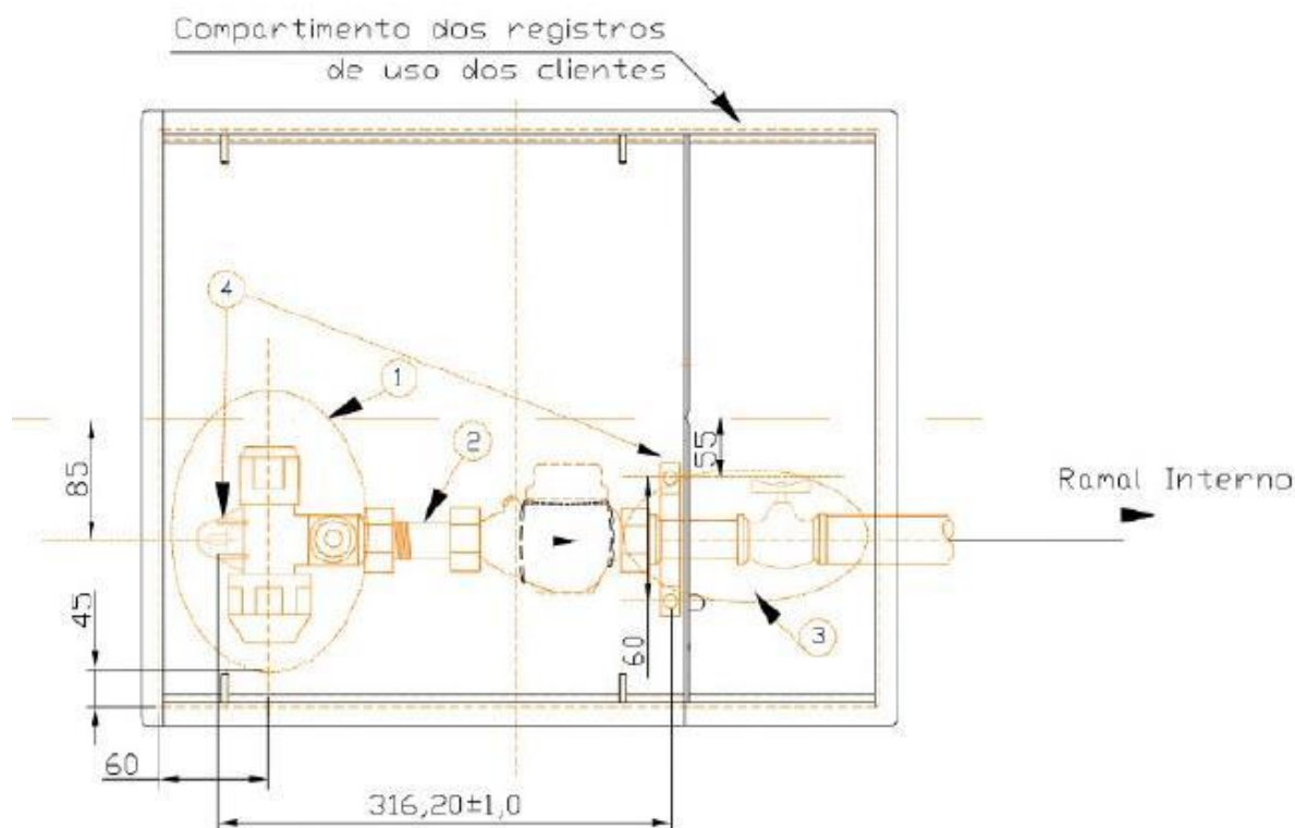
Figura 1 – Desenho esquemático de um dispositivo de medição
