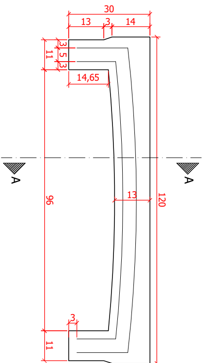
ELEVAÇÃO FRONTAL / GUIA CHAPÉU OBS: MEDIDAS EM CENTÍMETROS ESCALA: 1:10
