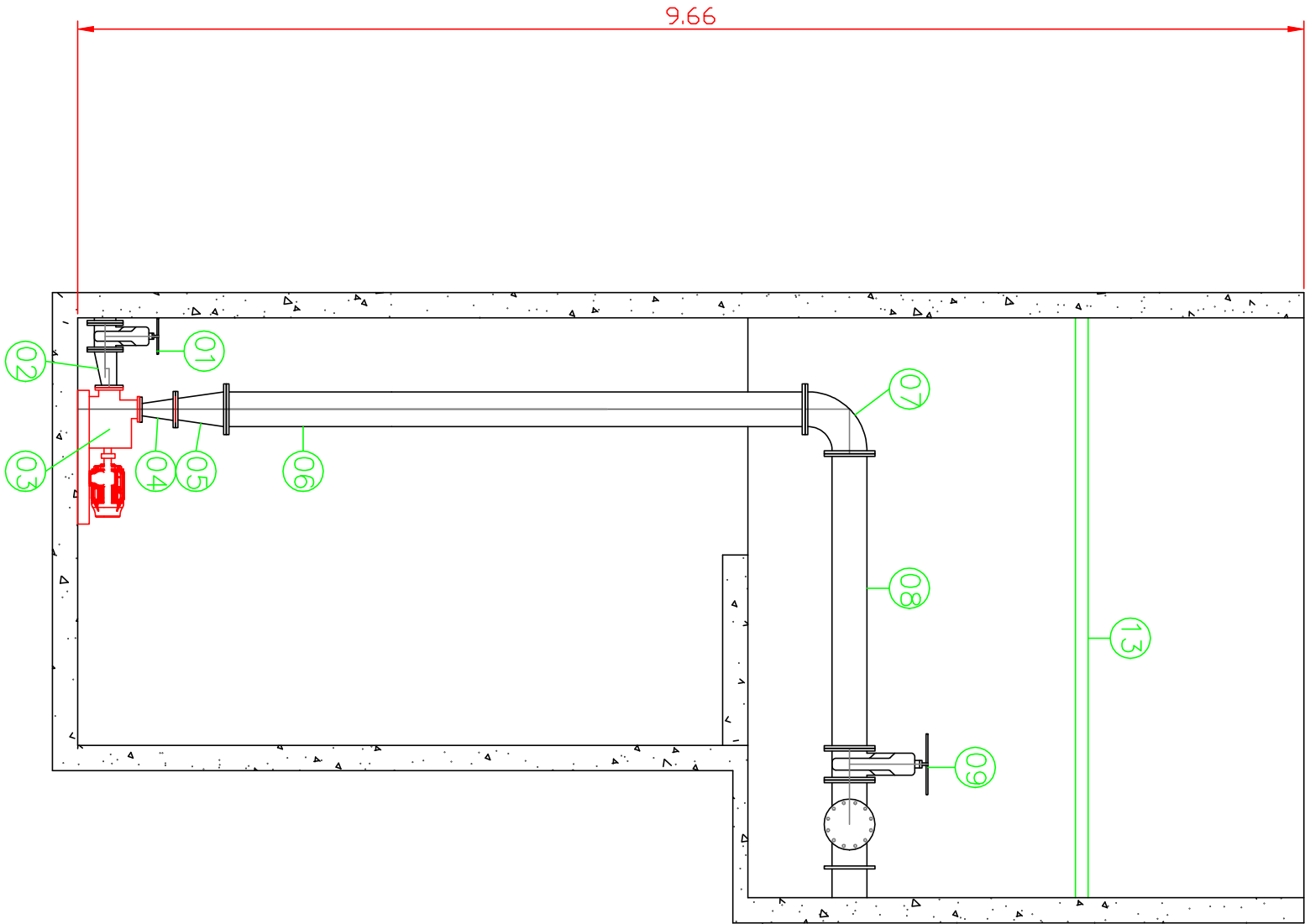
CORTE AA
