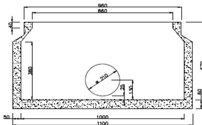
Corte AA
