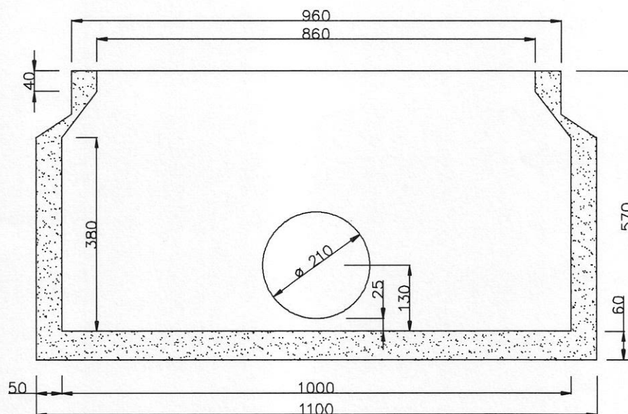
Corte AA
