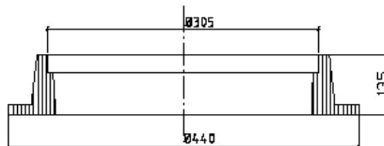
CORTE A-B
