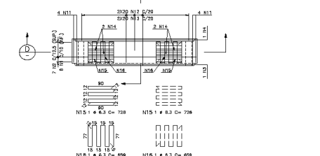
PLANTA SUPERIOR ESCALA 1:25
