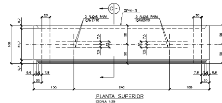
PLANTA SUPERIOR ESCALA 1:25
