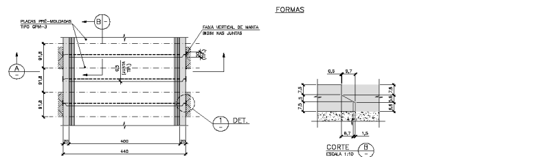
PLANTA PAREDES - DISTRIBUIÇÃO DAS PLACAS GPM-3 ESCALA 1:50
