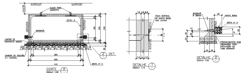
PLACA GPM-3 - (20X)
