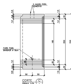
DETALHE 1 ESCALA 1:25
