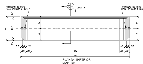
PLACA GPM-3 - (20X)
