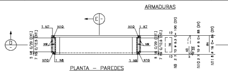
PLANTA - PAREDES ESCALA 1:25
