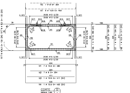
DETALHE 1 ESCALA 1:25
