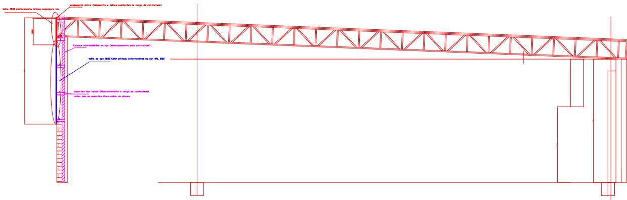
corte A-A
