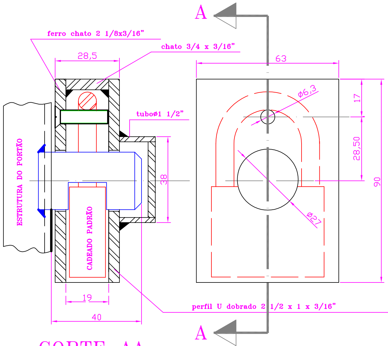
CORTE AA
