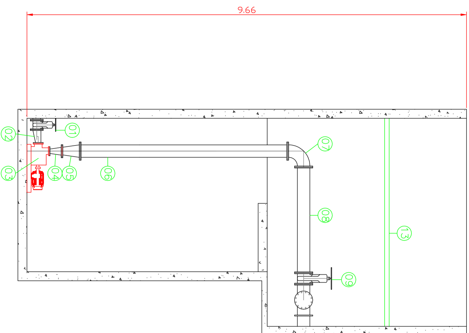
CORTE AA
